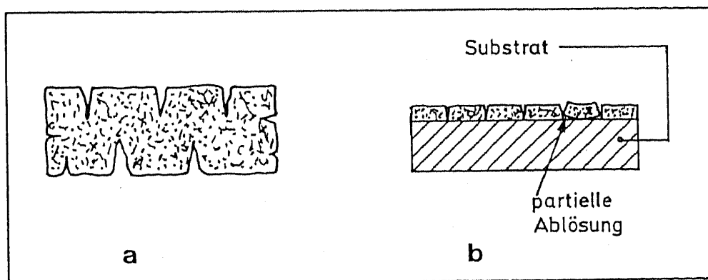
Bild 1. Schema einer typischen Trocknungsrißbildung bei einem kompakten Gel und bei einer Gel-Beschichtung
