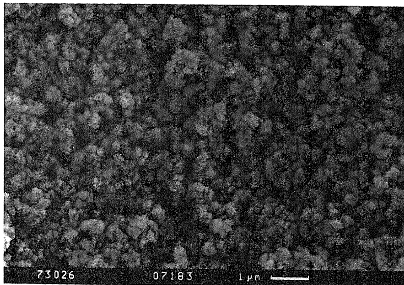
Bild 2. REM-Aufnahme von Aluminiumhydroxid mit globulärer Struktur; der Balken im Bild entspricht einer Länge von 1 µm
