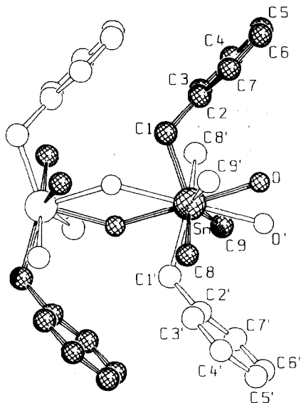
Abb. 1. Die "superpositionierte" Struktur in der Raumgruppe C_2 von Poly- \mu -hydroxo-benzyl-dimethyl-zinn ( A1Sn ). (Das eine "Individuum" ist vom anderen durch die Schraffur unterschieden.)
