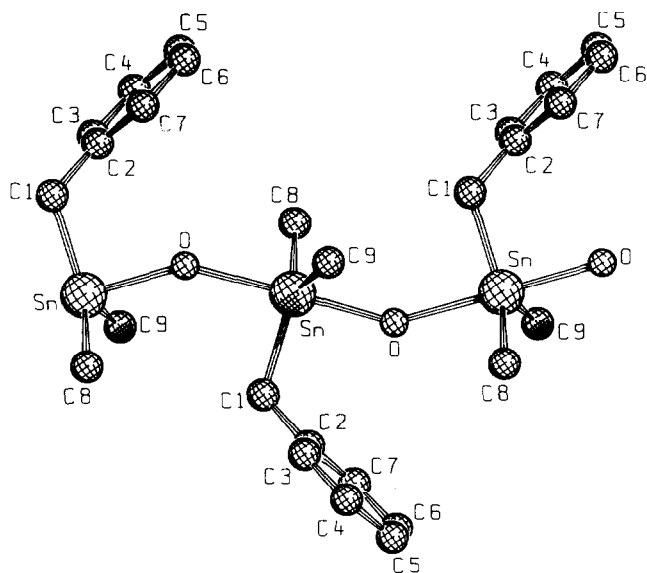
Abb. 2. Die "aufgelöste" Struktur von Poly- \mu -hydroxo-benzyl-dimethyl-zinn ( A1Sn ) (vgl. Text).
