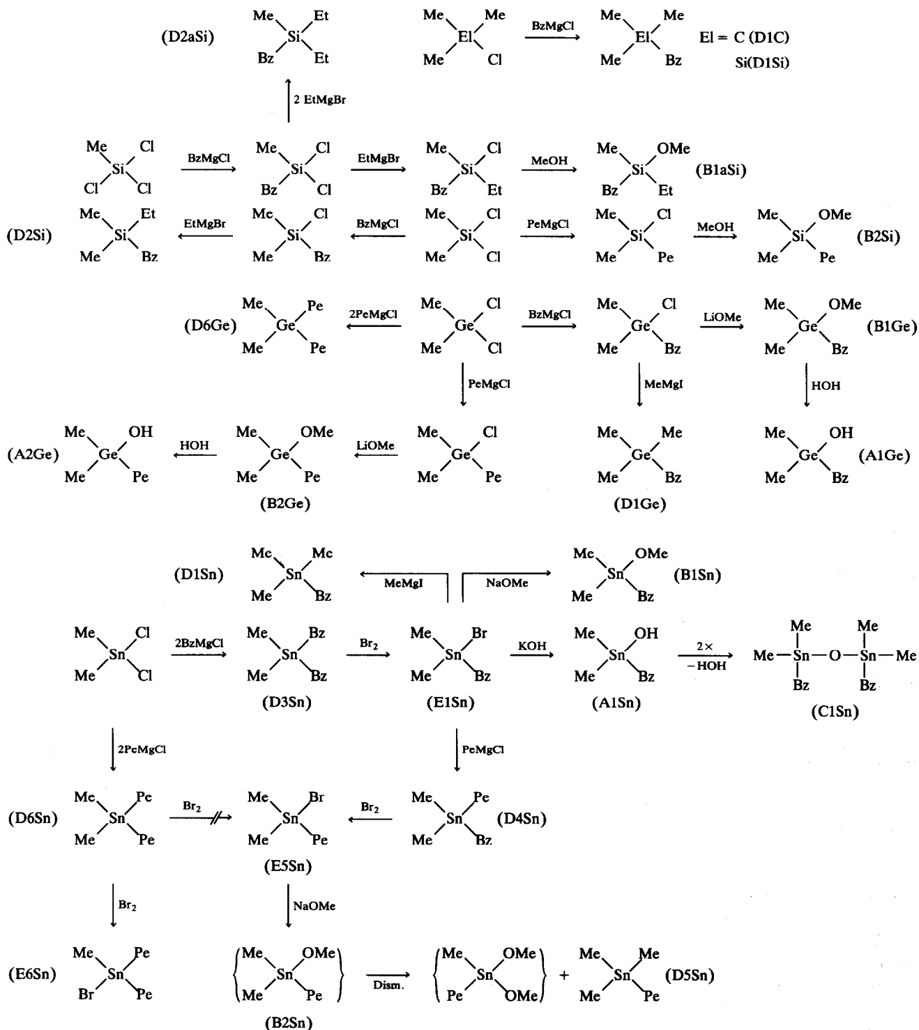
Schema 3. Zur Darstellung der homologen Verbindungen der Stoffklassen A bis E (Me = \text{CH}_3 , Et = \text{CH}_2\text{CH}_3 , Ph = \text{C}_6\text{H}_5 , Bz = \text{CH}_2\text{C}_6\text{H}_5 , Pe = \text{CH}_2\text{CH}_2\text{C}_6\text{H}_5 ).
