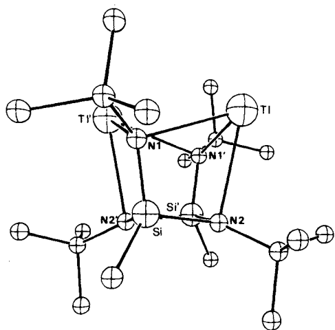
Abb. 3. Das Molekül 6 nach Röntgenstrukturanalyse (Die mit Strich markierten Atome ergeben sich aus den nicht markierten nach Anwendung der C_2 -Operation)
