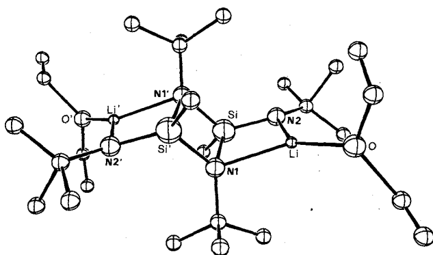
Abb. 2. Ansicht der „ trans -Verbindung“ 5b · [\text{Et}_2\text{O}]_2 .
