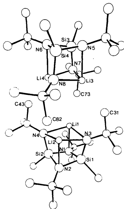
Abb. 1. Die beiden in der asymmetrischen Einheit der Elementarzelle befindlichen Moleküle 5a nach Röntgenstrukturanalyse
