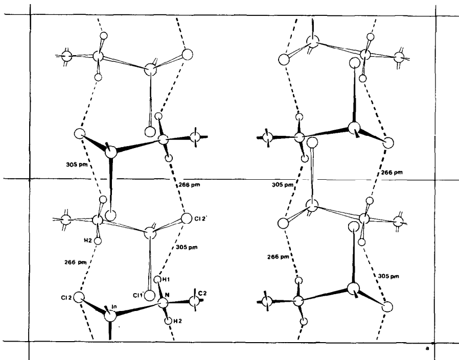
Fig. 1. Die Anordnung der Moleküle I im Kristall (Blickrichtung [0\bar{1}0] ). Die Methylgruppen sind der besseren Übersicht wegen nicht abgebildet. Die mit gleichartigen Bindungen gezeichneten Moleküle unterscheiden sich in ihrer Höhe um b/2 .
