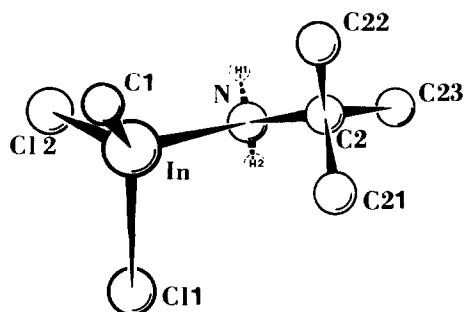
Fig. 2. Die Molekülstruktur von \text{MeInCl}_2 \cdot \text{H}_2\text{N}^t\text{Bu} (I) mit [0\bar{1}0] als Blickrichtung.
