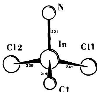
Fig. 3. Die Koordinationsfigur des Indiumatoms in I. An N und C(1) gebundene Atome sind weggelassen.
